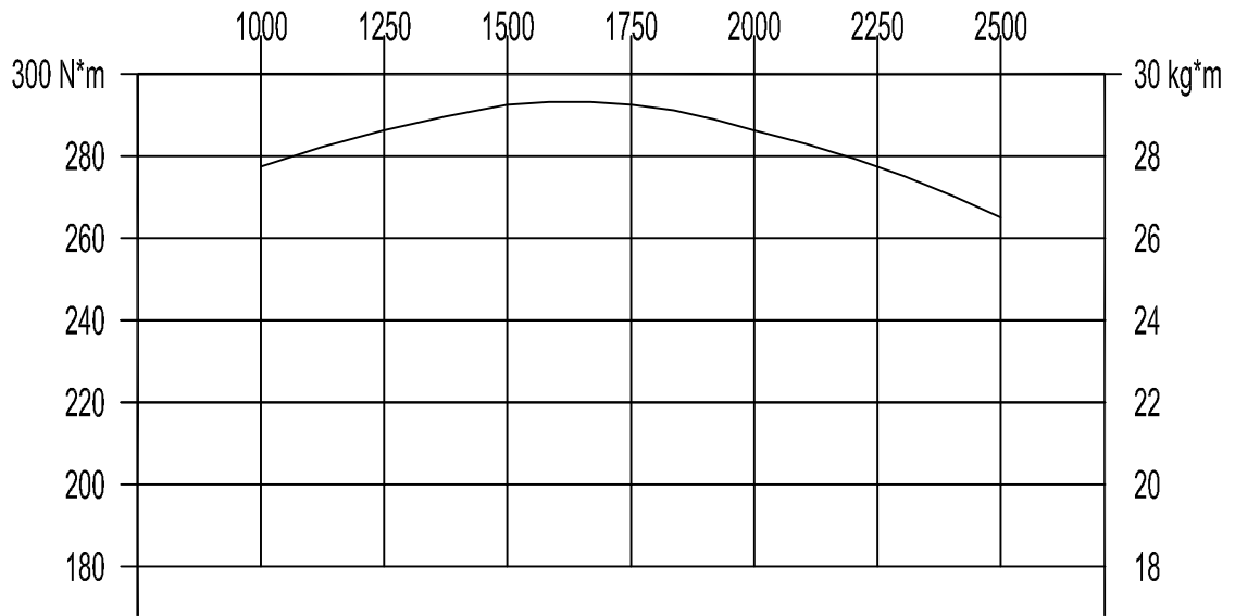
Par - Torque
