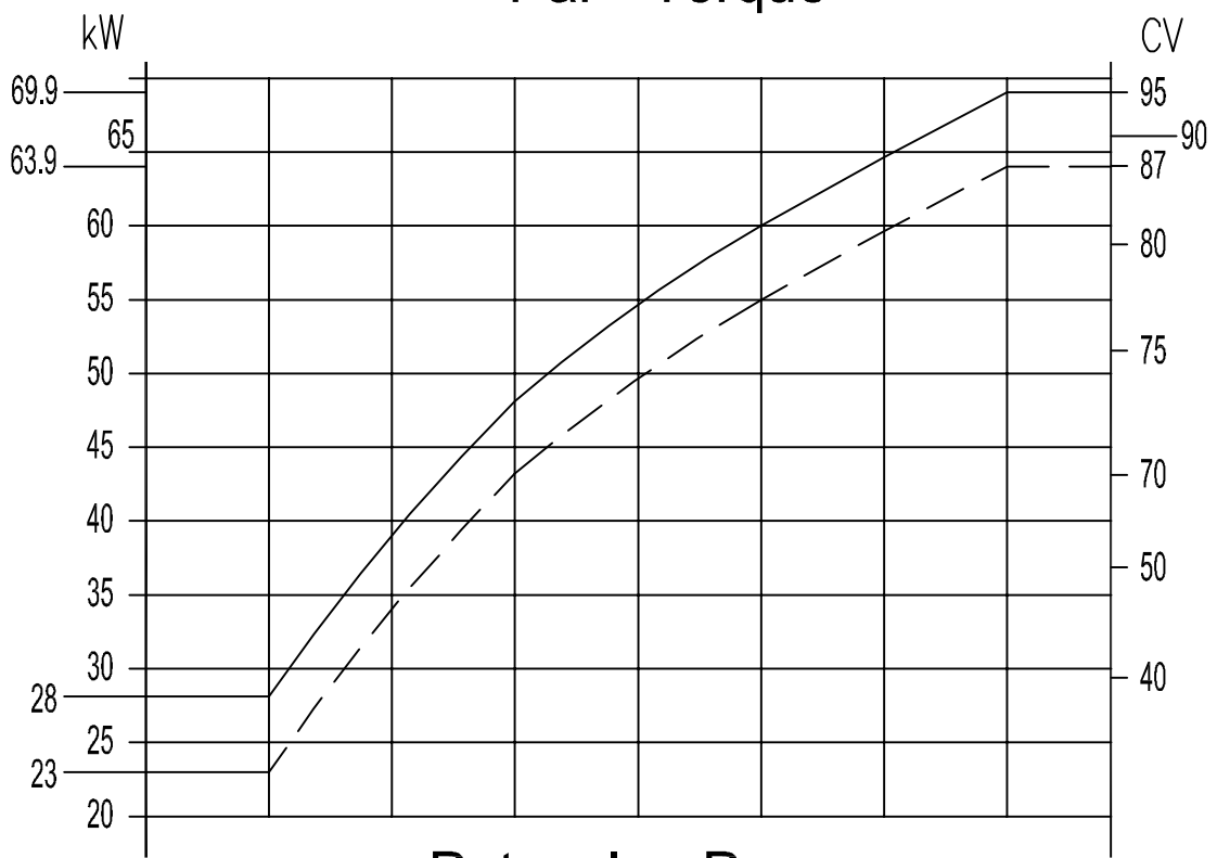
Potencia - Power
